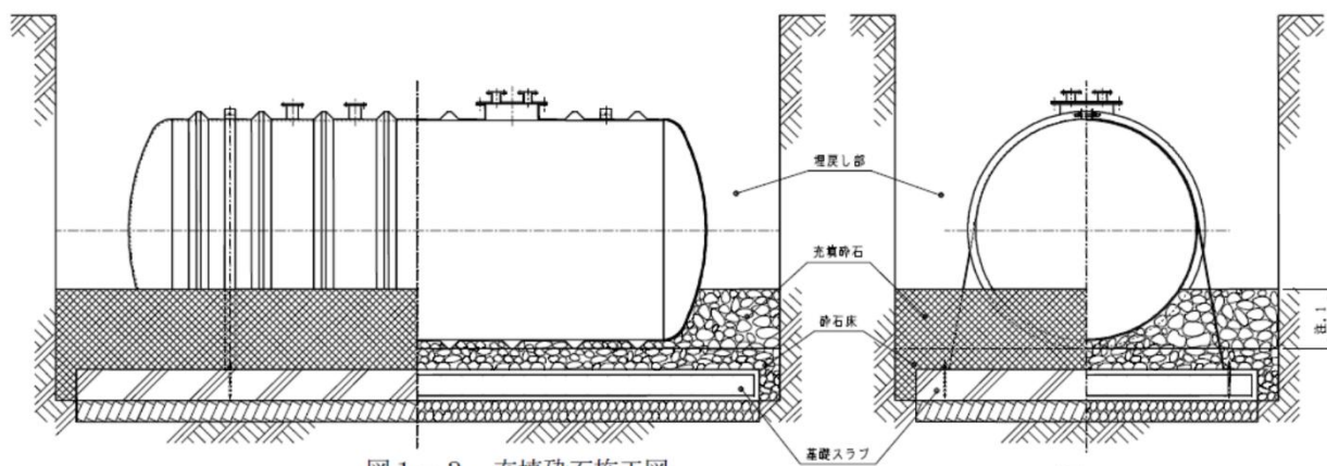
図1-3. 充填碎石施工図
