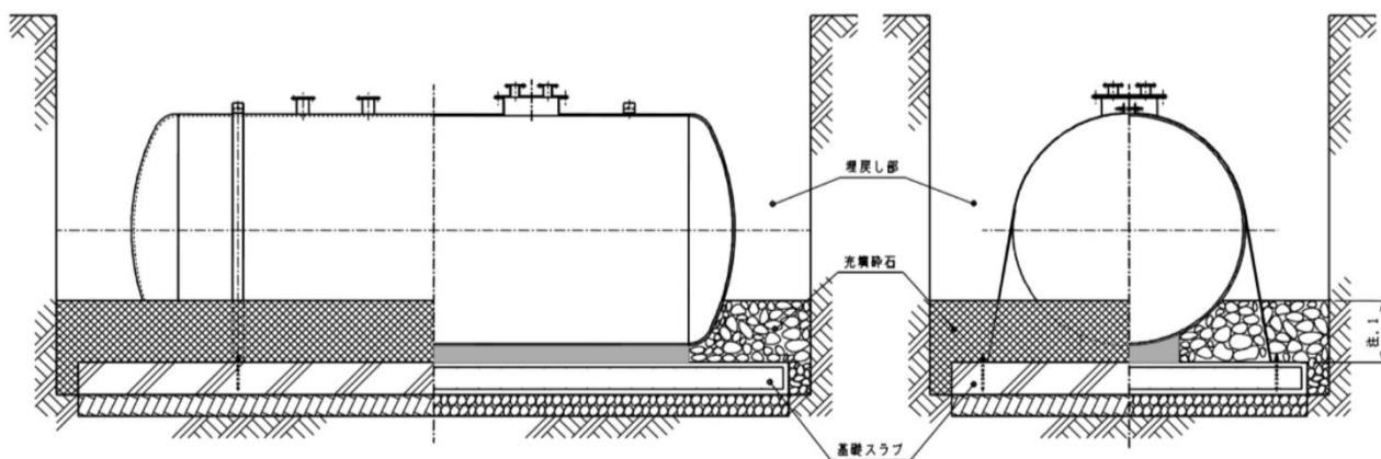
图 3-2. 充填碎石施工图
