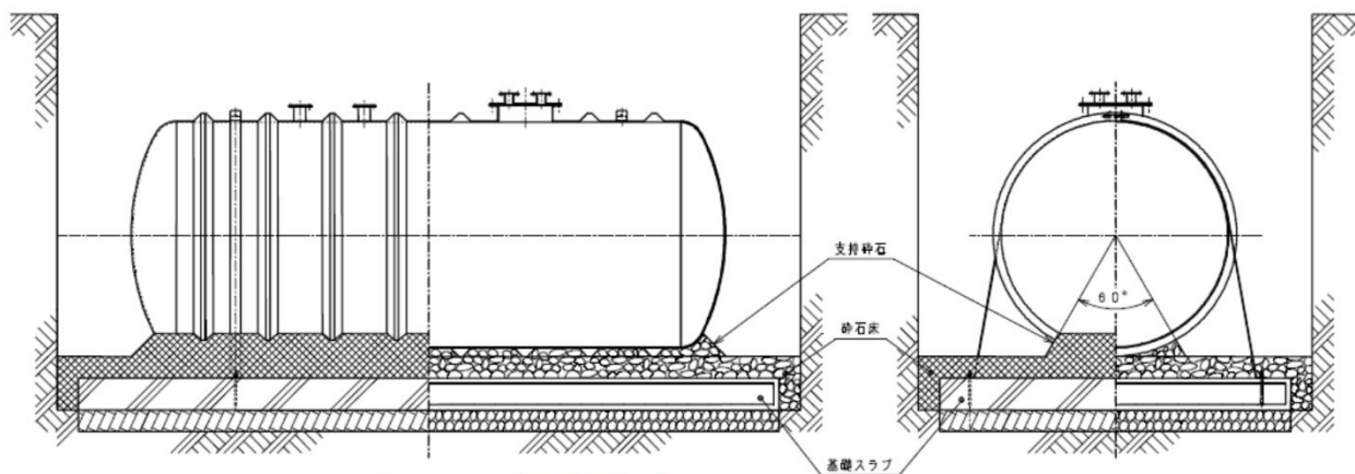
図1-2. 支持碎石施工図
