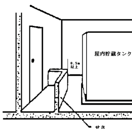
（せきを設ける例）
